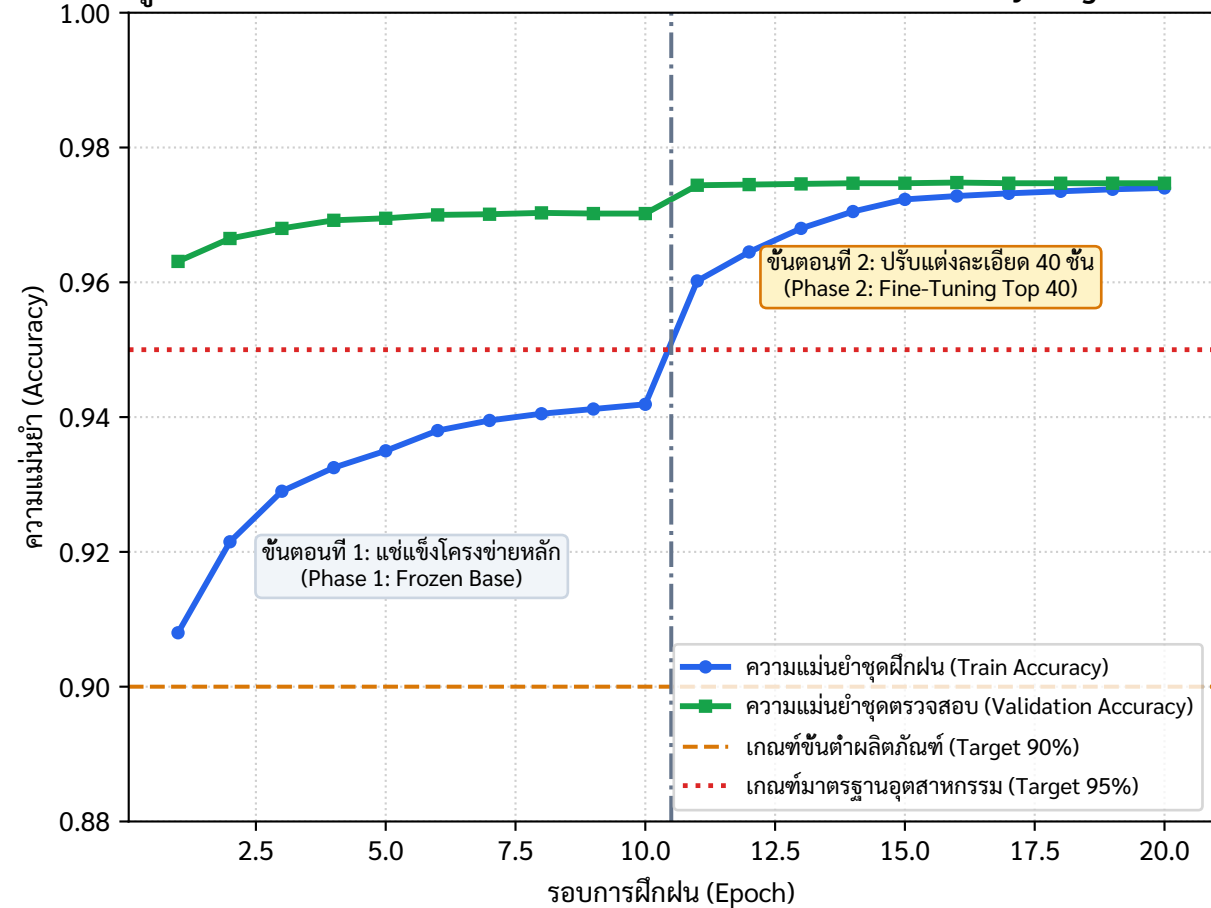
รูปที่ 3(a): ความแม่นยำตลอดการฝึกฝน 2 ขั้นตอน (Two-Phase Accuracy Progression)
