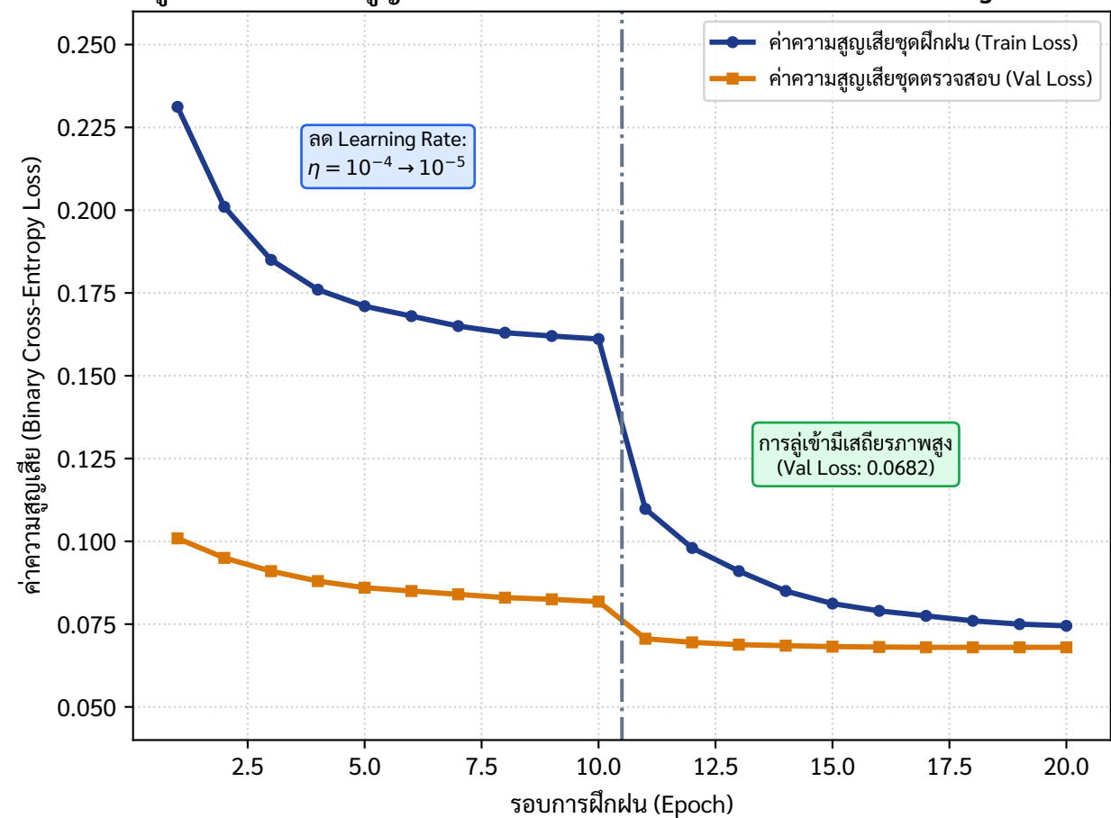
รูปที่ 3(b): ค่าความสูญเสียตลอดการฝึกฝน 2 ขั้นตอน (Two-Phase Loss Progression)
